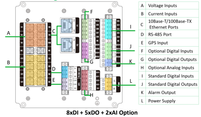
8xDI + 5xDO + 2xAI Option
